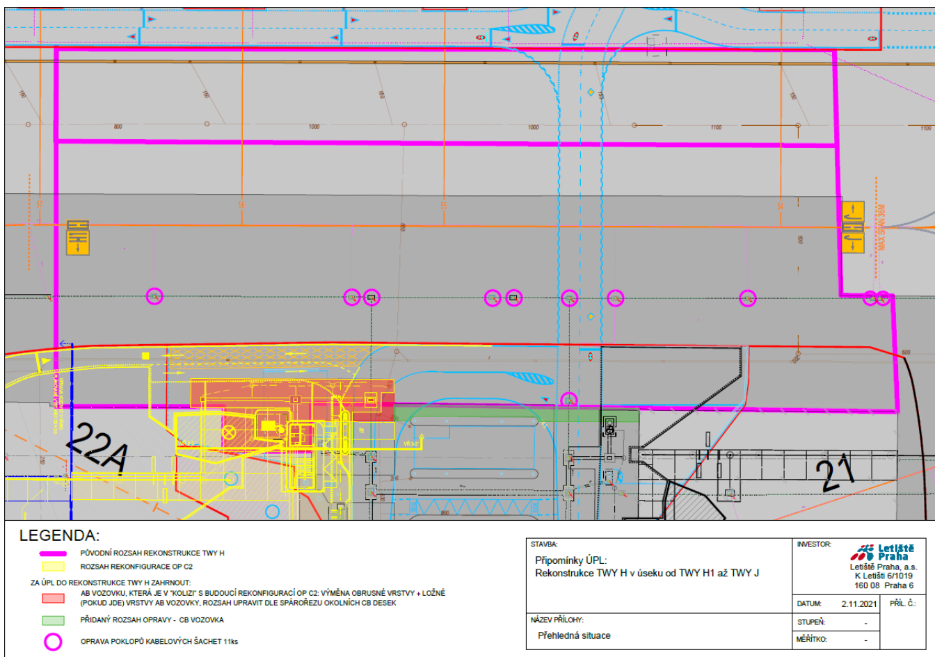
Obrázek č. 2 – situace – rozsah opravy plochy s AB krytem
